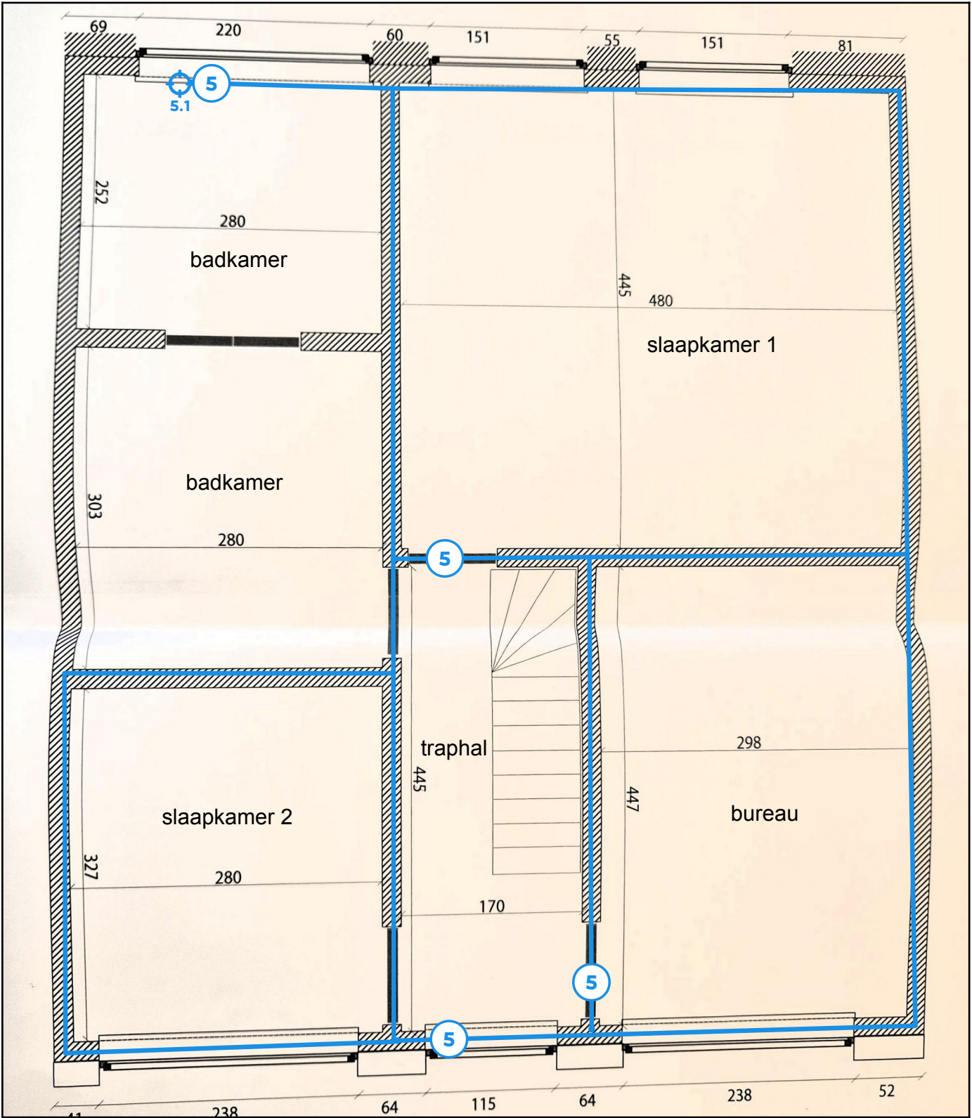
Legende van plan 1.5: Eerste verdiep pleisterwerk muren
