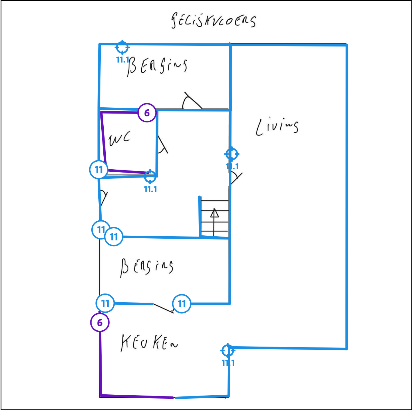
Legende van plan 1.1: Gelijkvloers pleisterwerk wanden Tegellijm wanden
