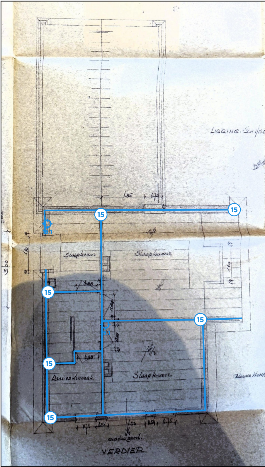
Legende van plan 1.5: Eerste verdiep pleisterwerk muren
